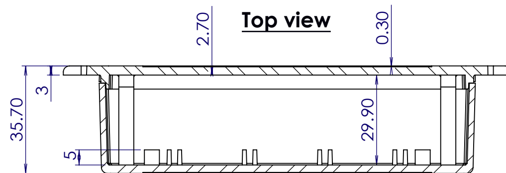
A-A Section
