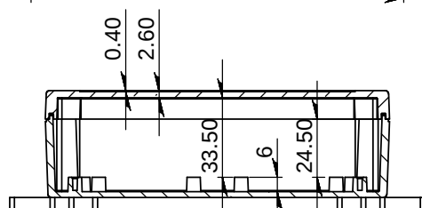
剖面圖 A-A
