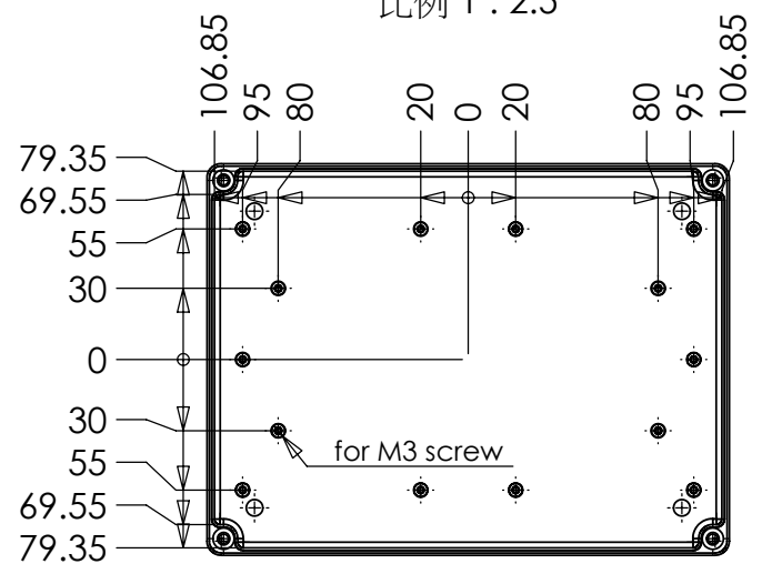
剖面圖 A-A 比例 1 : 2.5
