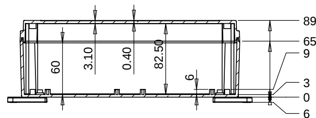
剖面圖 A-A 比例 1:3
